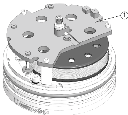
Abb. 1: Federgehäuse
