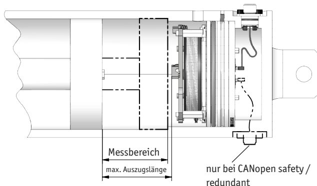
Abb. 2: Prüfung Auszugslänge
