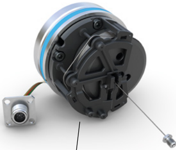
Druckfest bis 350 bar, Druckspitzen bis 450 bar Pressure-resistant up to 350 bar, Pressure peaks up to 450 bar
