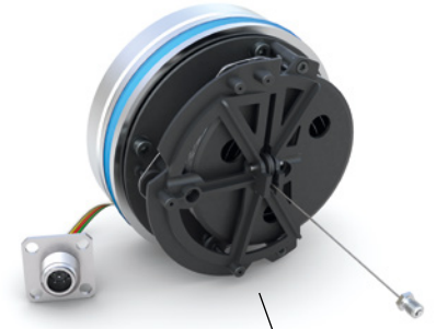
Messbereich bis 5 m Measurement range up to 5 m
