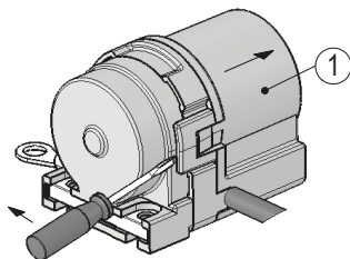
Abb. 4: Öffnen
