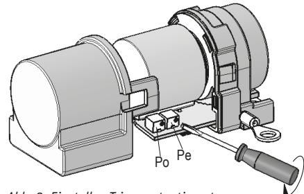
Abb. 8: Einstellen Trimpotentiometer
