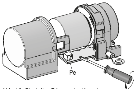
Abb. 10: Einstellen Trimpotentiometer
