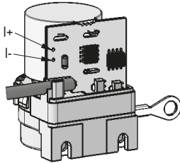
Abb. 6: Anschluss Potentiometer MWI
