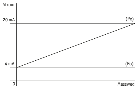
Abb. 9: Abgleich
