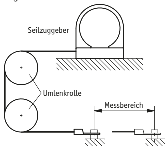
Abb. 3: Umlenkrolle
