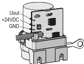
Abb. 7: Anschluss Potentiometer MWU
