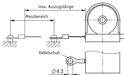
Abb. 2: Prüfung Auszugslänge
