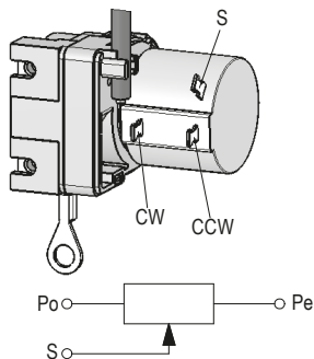
Abb. 5: Anschluss / Schaltbild Potentiometer
