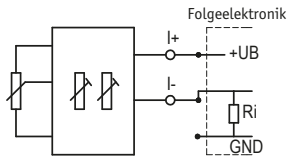
Abb. 6: Anschluss Potentiometer MWI
